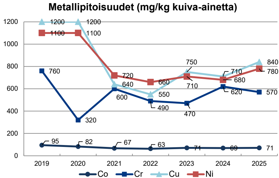
Kuva 2–1. Hiekanerotuskaivon hiekan Cr-, Cu- ja Ni-pitoisuudet vuosina 2019–2025.
