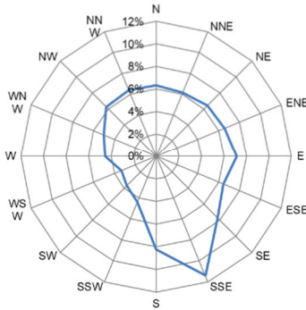
Kevitsa tuuliruusu, 8.5.-6.6.2025
