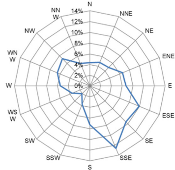
Kevitsa tuuliruusu, 1.-15.8.2025
