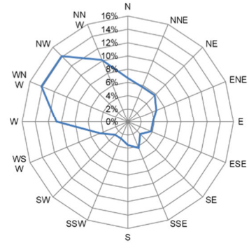
Kevitsa tuuliruusu, 14.3.-11.4.2025
