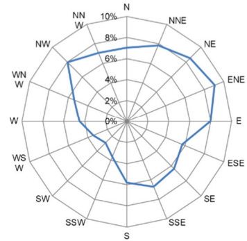
Kevitsa tuuliruusu, 7.6.-27.6.2025
