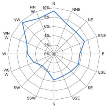
Kevitsa tuuliruusu, 28.6.-18.7.2025
