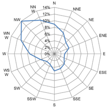
Kevitsa tuuliruusu, 12.4.-8.5.2025
