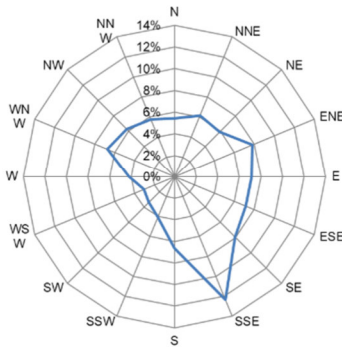
Kevitsa tuuliruusu, 19.7.-31.7.2025
