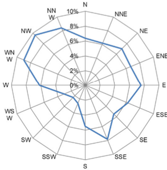
Kevitsa tuuliruusu, 16.1.-12.2.2025
