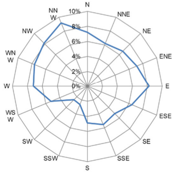
Kevitsa tuuliruusu, 16.12.2024-15.1.2025
